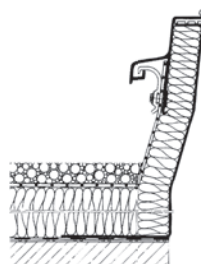
Sistem soclu metalic tip RAK, cu înălțimea de 40 cm cu sistem de prindere pe acoperiș OPTIMAL
