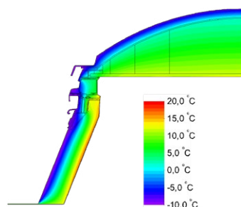
Curbă izotermă TOP-90 Plus
